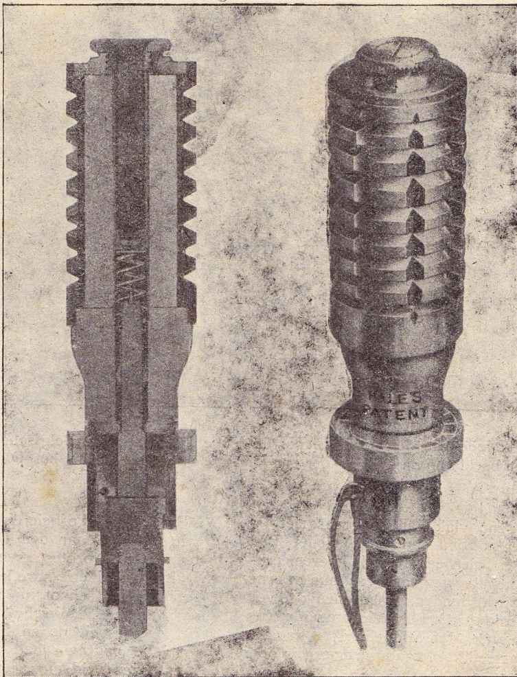
Doorsnede en aanzicht van een Engelsche handgranaat.
