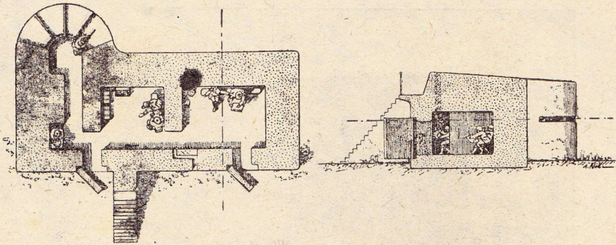
Plattegrond en zij-aangezicht van een der beruchte Duitsche zoogenaamde Pillendozen in Vlaanderen.
